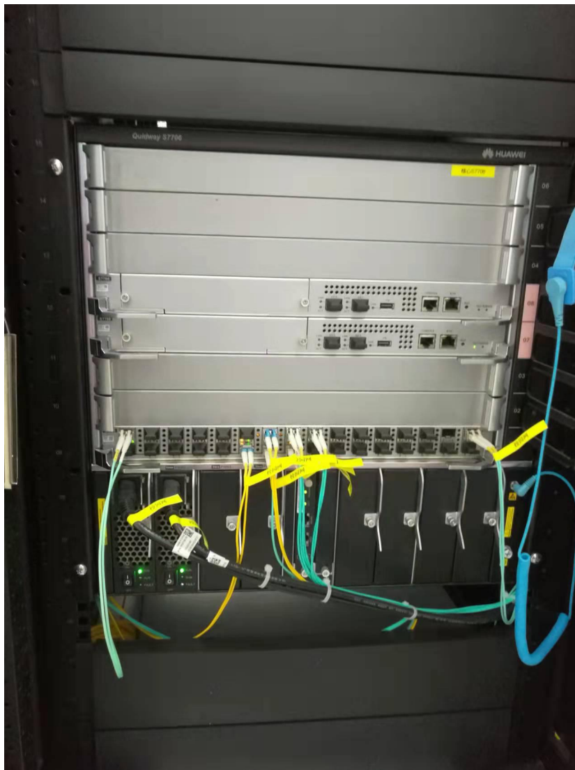
图 1 核心交换机（华为 S7706）
